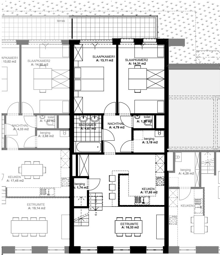
NIVEAU 1
